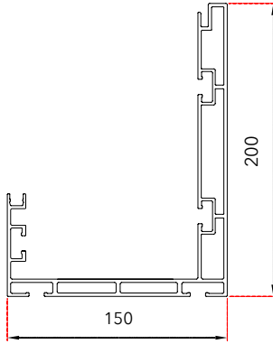
Side View Yandan Görünüş
