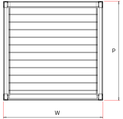
Top View System Closed Üstten Görünüş Sistem Kapalı
